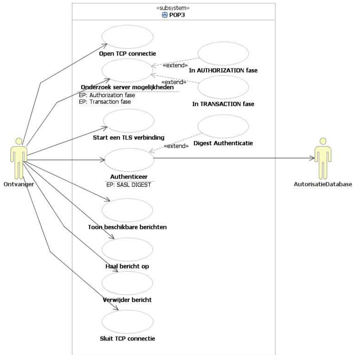
Figuur 1: Interactie tussen gebruiker er POP3-server bij gebruik van SASL
